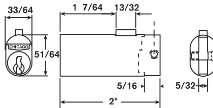
5002-LP DK-P-1 key blank
